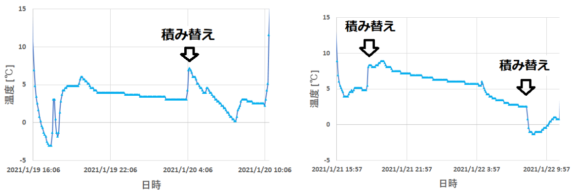
図3 実証実験の結果。大阪から東京への低温物流において、一部を除いて、温度が維持されている。
